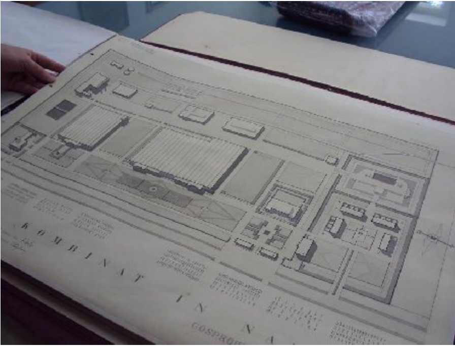
Fabrikanın yerleşim planı
